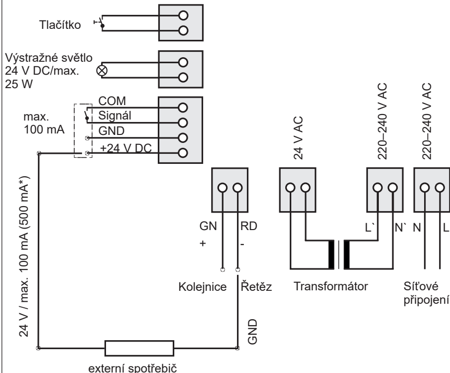
Obr. Plán připojení Stropní řídicí systém
